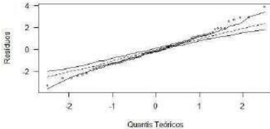
Figura 3 – Gráfico de quantis normais com envelope simulado para o modelo de regressão Poisson com função de ligação raiz quadrada.
